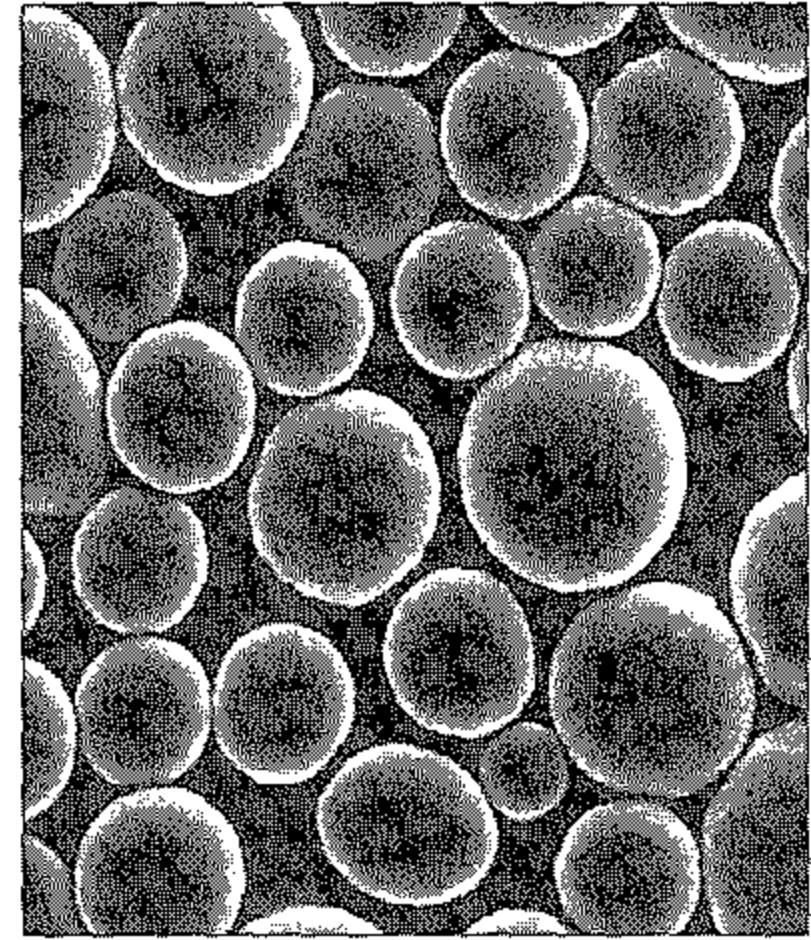
Spezieller Kugeltoner mittlerer Durchmesser 7-9 \mu\text{m}
