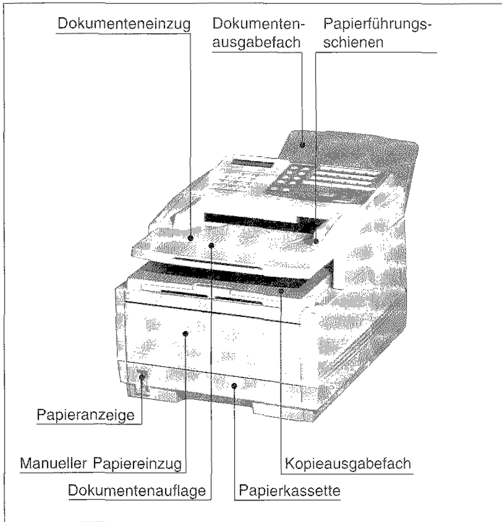
Vorderansicht
